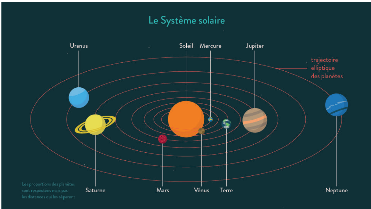
Le système solaire
